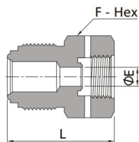
Переходник понижающий с наружной на внутреннюю резьбу
