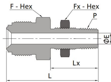
Переходник проходной с наружной цилиндрической резьбы на наружную NPT (с гайкой для монтажа)
