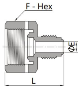
Переходник понижающий с внутренней на наружную резьбу
