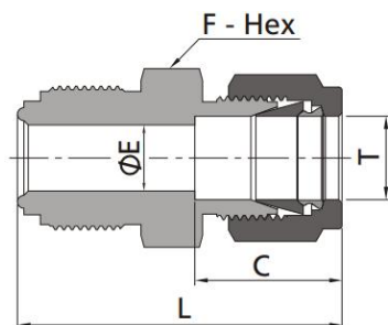
Переходник с наружной цилиндрической резьбы на трубный фитинг
