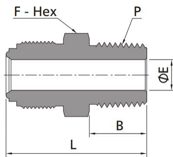
Переходник с наружной цилиндрической резьбы на наружную NPT
