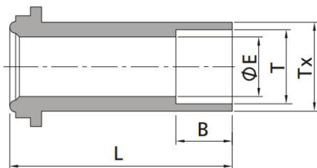
Втулка под сварку в раструб с длинной дюймовой трубкой
