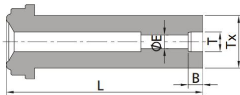
Понижающий ниппель под сварку втруб
