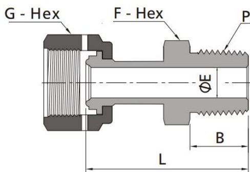
Переходник с наружной гайки на втулку с внешней резьбой NPT
