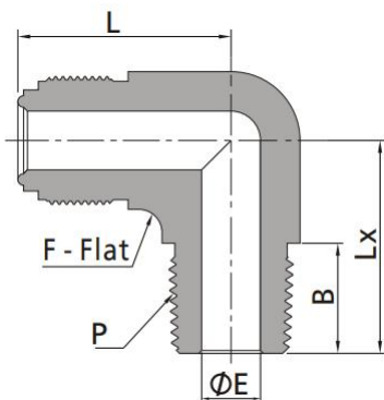
Переходник угловой с наружной цилиндрической резьбы на наружную NPT
