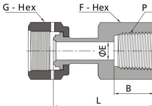
Переходник с наружной гайки на втулку с внутренней резьбой NPT
