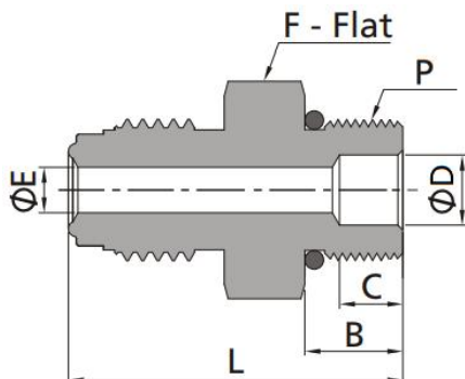
Переходник с наружной цилиндрической резьбы на наружную SAE/MS
