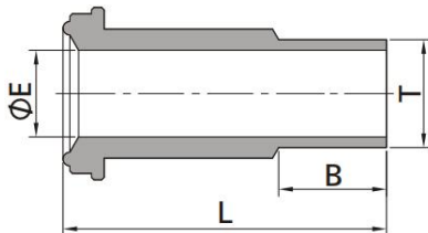
Втулка под приварку вставной
