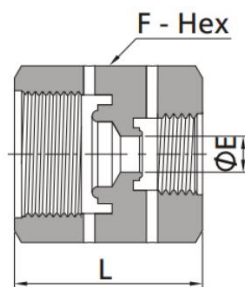
Муфта понижающая с внутренней резьбой
