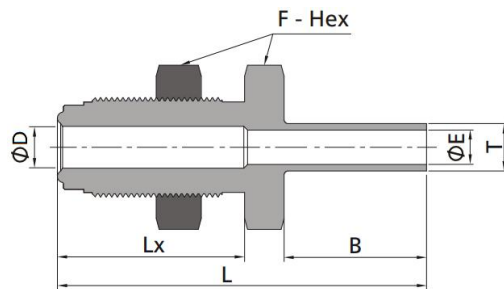
Переходник проходной с наружной резьбой под приварку (с гайкой для монтажа)
