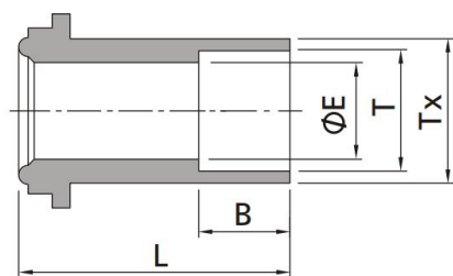
Втулка под сварку в раструб с короткой дюймовой трубкой
