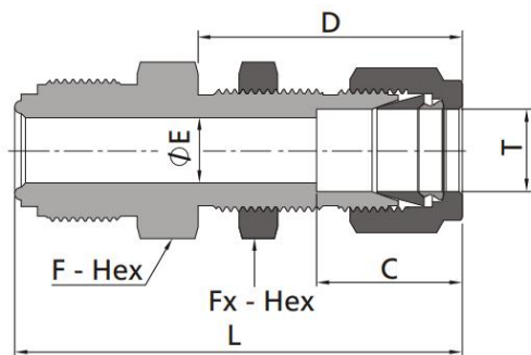
Переходник проходной с наружной цилиндрической резьбы на трубный фитинг (с гайкой для монтажа)
