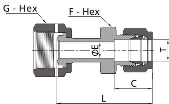
Переходник с наружной гайки на трубный фитинг
