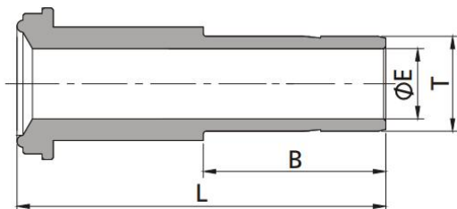
Втулка с трубным адаптером
