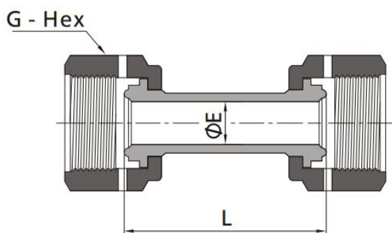
Муфта с двумя наружными гайками
