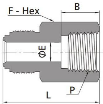
Переходник с наружной цилиндрической резьбы на внутреннюю NPT
